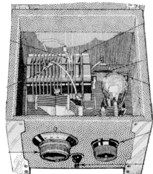
Aufbau des Kurzwellenvorsatzes von Elex.
