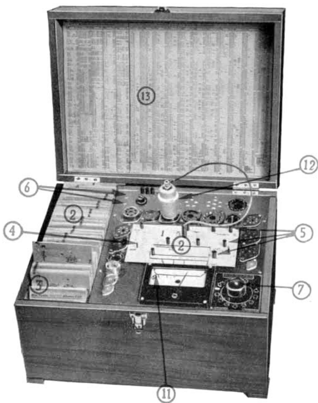
Modell W 19 mit aufgelegter Prüfkarte
