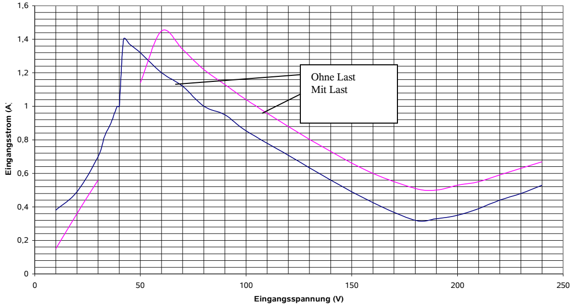
Stromaufnahme im Leerlauf und mit 40-W-Glühlampe als Last
