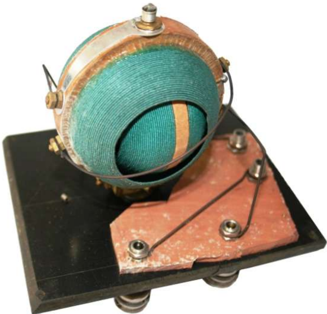
ROSENMAYR Detektorapparat, Innenaufbau mit Kugelvariometer
