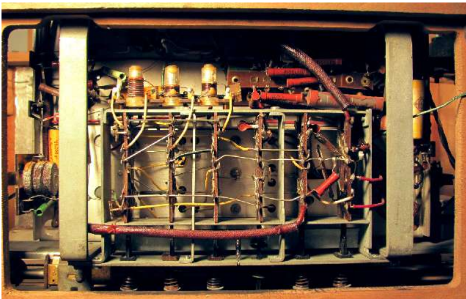
INGELEN Genius, Ansicht von unten
