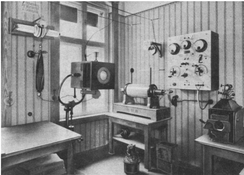
Abb. 2 Das Röntgenlaboratorium des Verfassers zur Unter- suchung von Radioröhren
