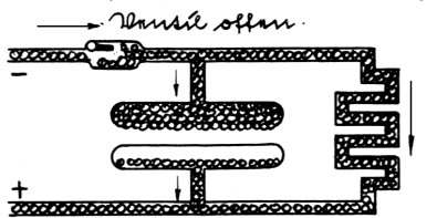
Abb. 6. Die Elektronenbewegung im Stadium 1. Der Kondensator wird durch einen Stromstoß aufgeladen, während dieser Zeit fließt ein Teil des von links herkommenden Stromes natürlich auch über unsern Widerstand.
