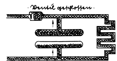
Abb. 7. Die Elektronenbewegung im Stadium 2. Das Ventil ist geschlossen. Der Kondensator entlädt sich deshalb nur nach rechts u. schießt so auch ohne die äußere Spannung einen Strom durch den angeschlossenen Widerstand.
