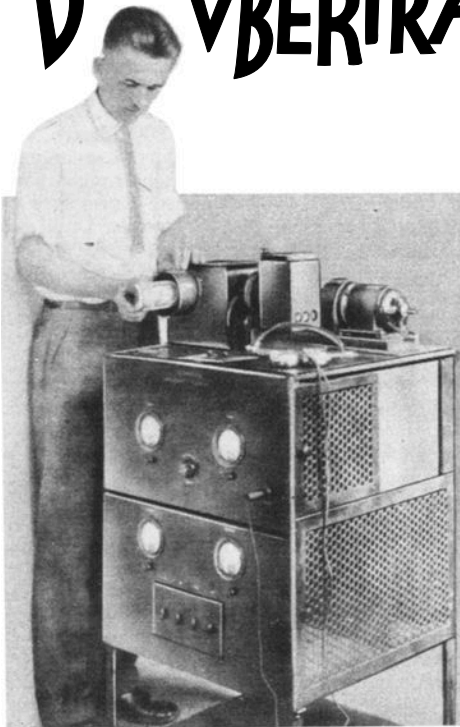
Der Sende-Apparat
