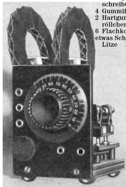
Abb. 2. Das Gerät betriebsfähig
