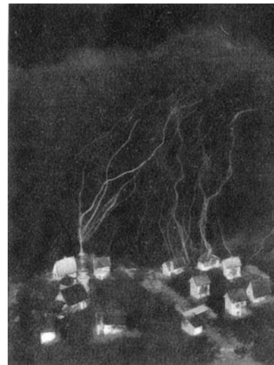
Abb. 4. Modellversuche über Blitzentladungen.
