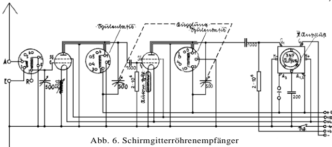
Abb. 6. Schirmgitterröhrenempfänger
